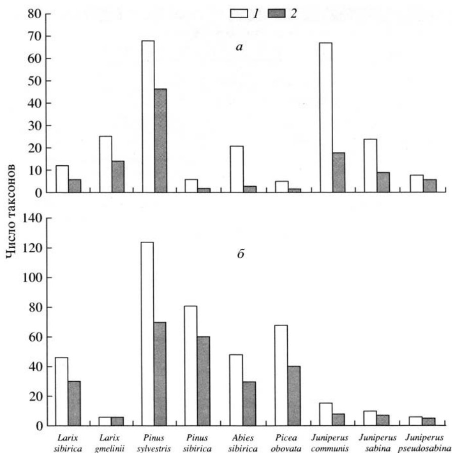
Рис. 1. Характеристика синонимии видов хвойных: а - согласно данным [1, 12] (общее число таксонов вида - 1, в том числе видового ранга - 2); б - по базе данных (общее число таксонов вида - 1, без учета синонимов - 2).
