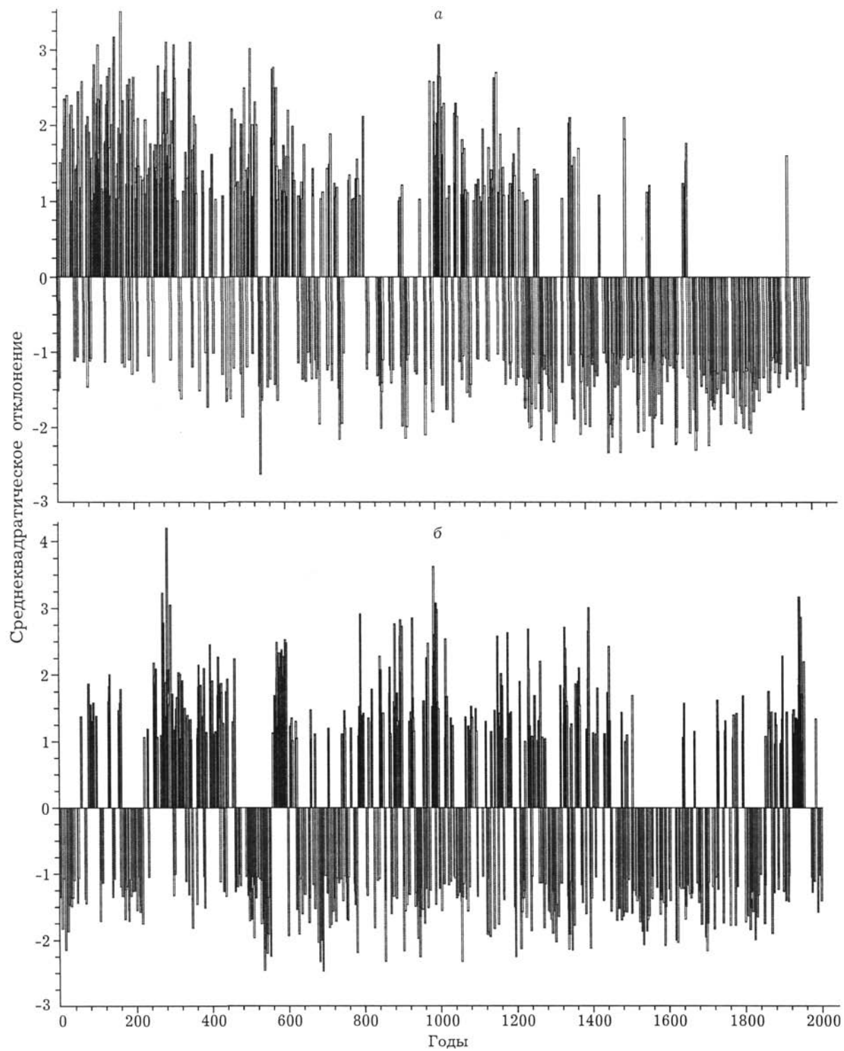
Рис. 1. Теплые и холодные годы, зафиксированные в длительных древесно-кольцевых хронологиях: а - по Индигирке, б - по Таймыру.
