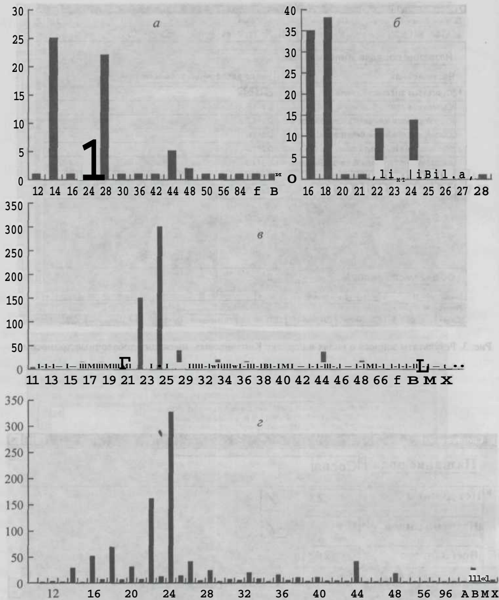
Рис. 5. Гистограммы распределения чисел хромосом различных классов отдела голосеменных. a — гнетовые; б — сикадовые; в — хвойные; г — весь отдел голосеменных растений. По оси абсцисс — число хромосом, по оси ординат — число видов. А — анеуплоиды, В — добавочные хромосомы, М — миксоплоиды, X — химеры, f — фрагменты.
